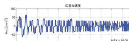
免震効果データ (応答計算)
