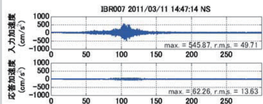
免震効果データ (応答計算)
